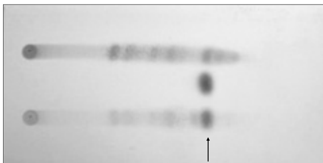
写真2 グラヤノトキシンのTLCクロマトグラム 上段: ハクサンシャクナゲ葉の試験溶液, 中段: グラヤノトキシンI, 下段: 試験溶液 左から右に展開(右端が溶媒先端)
